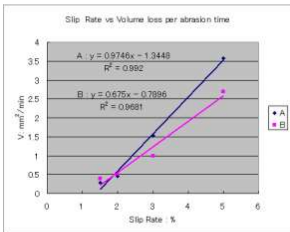
スリップ率 VS 摩耗体積
