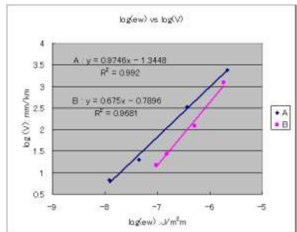
1000km 当りの摩耗量 VS 摩耗エネルギー
